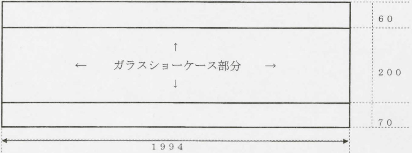
① ギャラリー、正面から見た図 (単位: cm)
