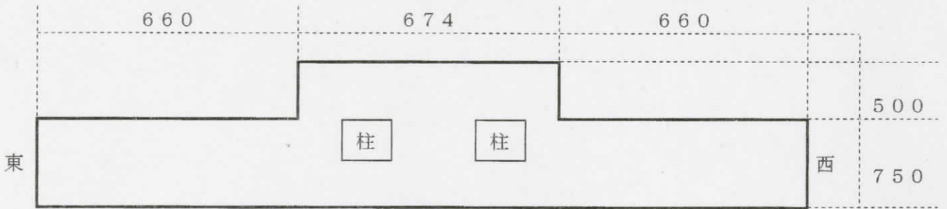
② ギャラリー、真上から見た図 (単位: cm)
